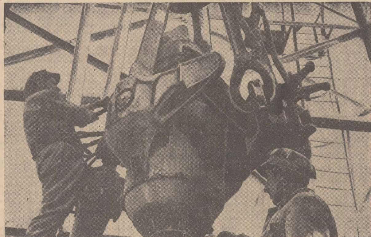
Se repară capul hidrolic la o sondă în foraj.
