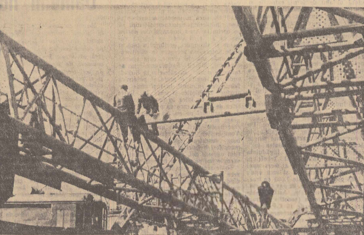
Instalație de foraj 4 LD, produsă de uzinele „I. Mai”-Ploiești
