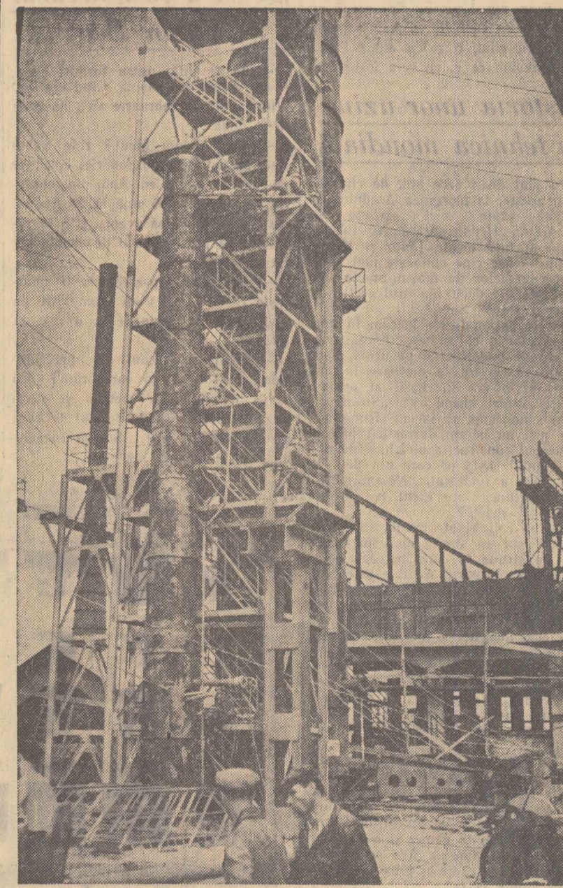
Rafinăria nr. 10 Onești își dezvoltă activitatea prin construirea și punerea în funcțiune a noi instalații moderne în clîșeu. Una din cele două instalații de cracare catalitică în curs de montaj.
