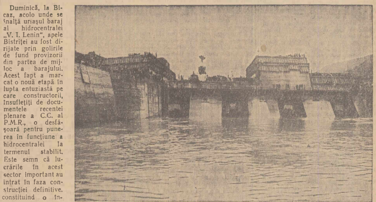
Trecerea apelor Bistriței prin golirile provizorii de fund ale barajului, după închiderea canalului de deviere. Foto: AGERPRES
