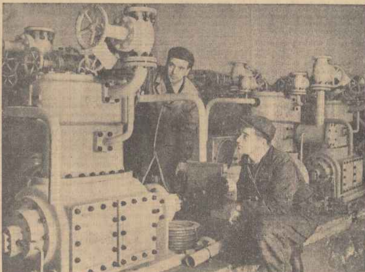
Uzinele „Tehnofrig” din Cluj au devenit bine cunoscute pentru variatele tipuri de mașini fabricate pentru indus- tria alimentară. În cișcu: Controlorul tehnic Francisc Baki și maistrul Carol Debeliyak fac ultima verificare com- presorului destinat instalațiilor frigorifice.
