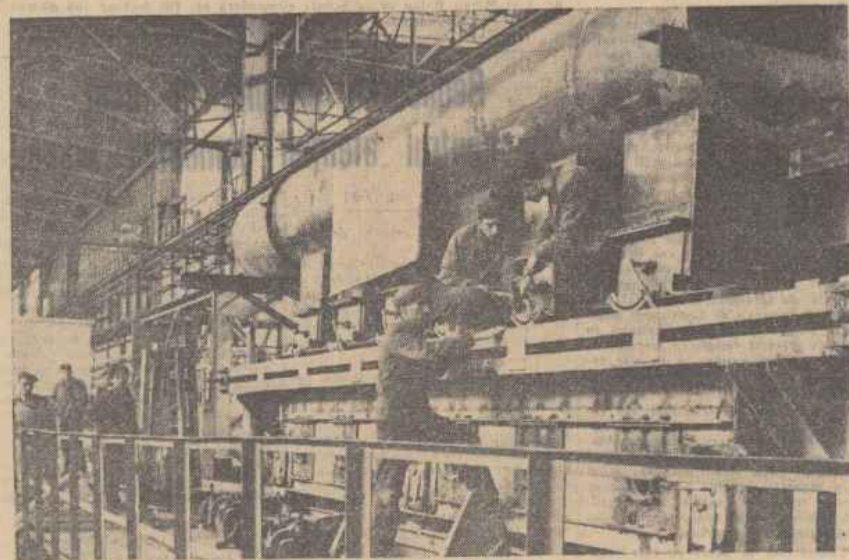
Se lucrează la montajul celui de-al doilea cuplor al laminorului de 650 mm. de la Hunedoara.
