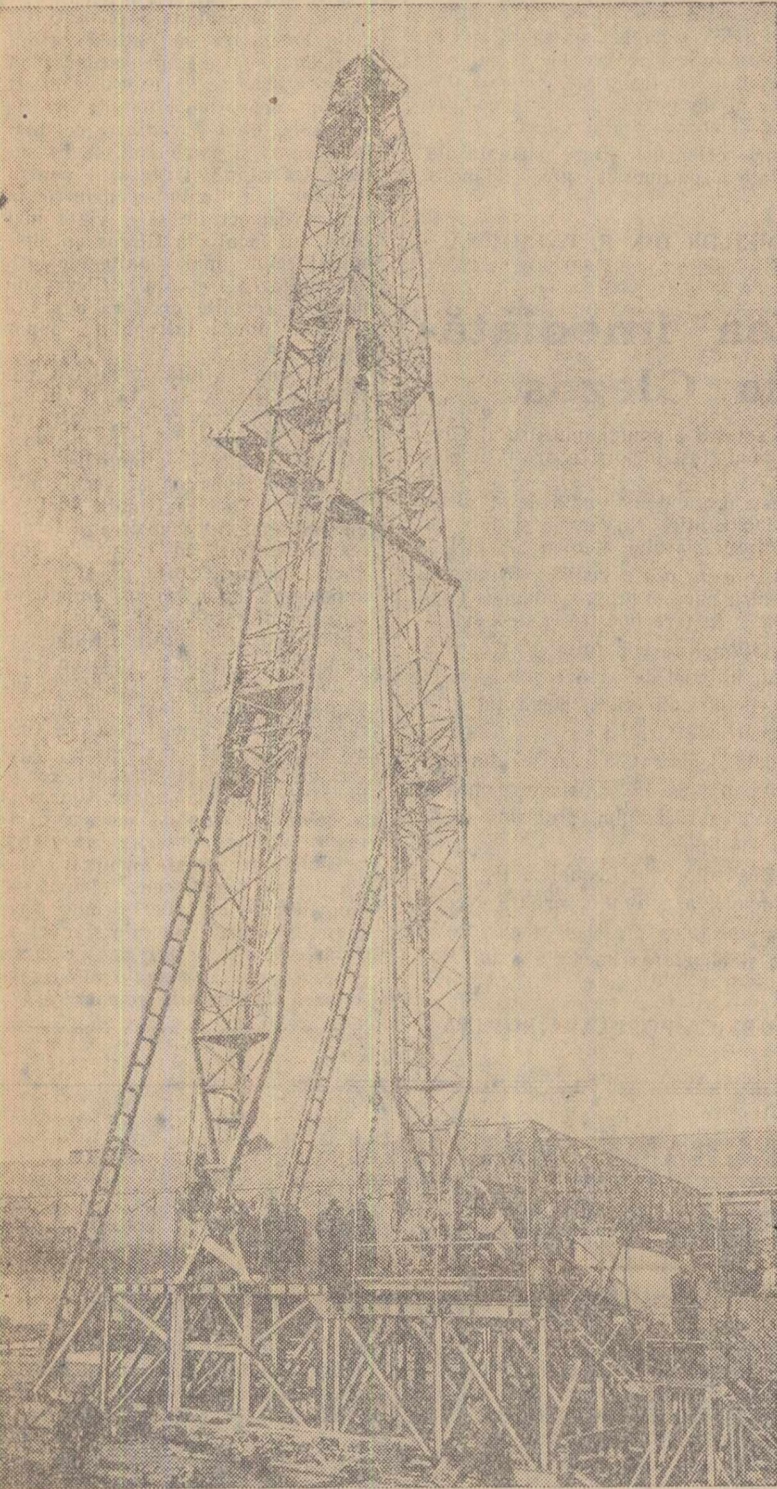
Instalație de foraj 4-LD, pentru săparea sondelor
