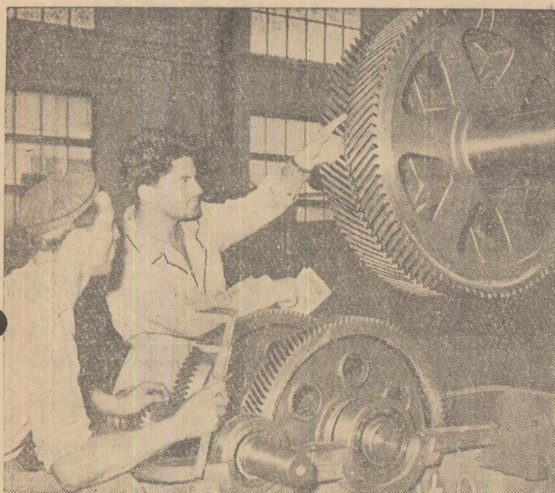
Brigada lui Vasile Pană de la Uzinele „Mao Tze-dun” din București lucrează reductoare pentru morile de ciment — piese de mare tehnicitate. În cinstea zilei de 23 August, brigada a dat două reductoare peste plan. În clișeu: Ing. Romeo Vircolici, verificând împreună cu șeful brigăzii, Vasile Pană, calitatea reductoarelor din lotul pentru R. P. Chineză. Foto: A. CONSTANTINESCU
