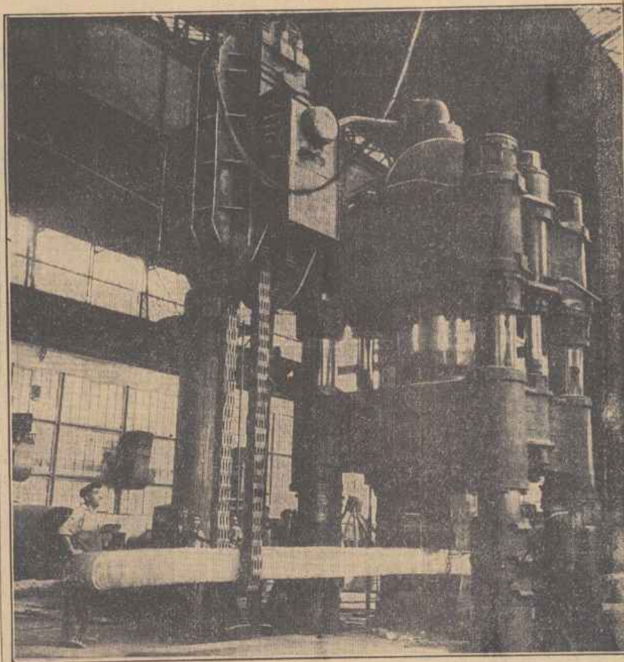
De câțiva ani, uzinele „Progresul” din Brăila au început să fie cunoscute în țară prin diversele utilaje și mașini pe care le fabrică. Vă prezentăm azi un aspect din munca metalurgistilor acestei întreprinderi. Cliseul de mai sus reprezintă un colț din secția forje grele a uzinei „Progresul”. Urașă presă de 2.500 tone care se vede în cliseu este condusă cu precizie de echipa lui Iordan Dragomir. Lingurile grele de metal abia scoase din cuptor sunt presate cu ușurință de acest agregat puternic. Foto: NICU VASILE
