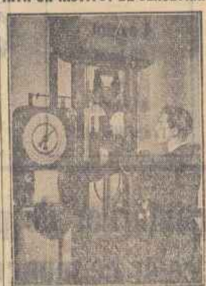
Institutul de cercetări chimice din Capitală aduce un aport valoros la realizarea unor noi și importante produse chimice. În laboratorul de cercetări fizico-mecanice al Institutului, preparatorul Liviu Ionescu determină rezistența la tracțiune a unui material plastic. Foto AGERPRES
