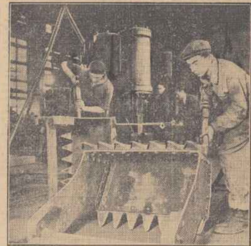
Colectivul Atelierele centrale de reparaii „Nuftra Dezideriu” din Baia Mare, aduce un important aport la buna desfășurare a muncii în minele din regiune. Cliseul de mai sus prezintă un aspect din secția lăcătugerii a atelierele. Aci se execută cupe pentru escavatoarele din mină cu ajutorul cărora se încarcă minele în vagoane.
