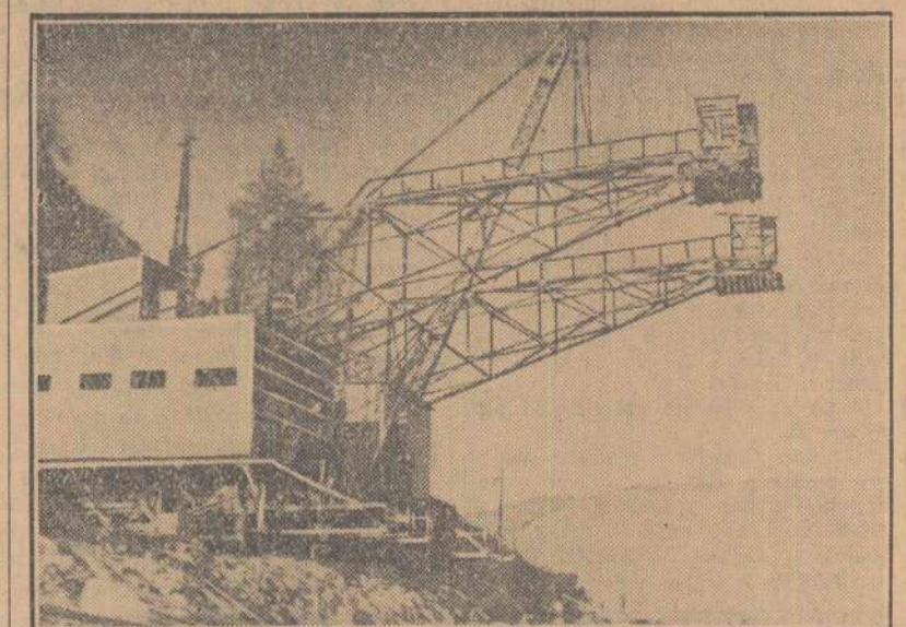
Pe malul Bistriței, în sectorul barajului hidrocentralei „V. I. Lenin” de la Bicaz, au fost aduse numeroase mecanisme de înaltă tehnicitate. În cliseu: Turnurile macaralei funicular care va transporta betonul la locul turnării.
