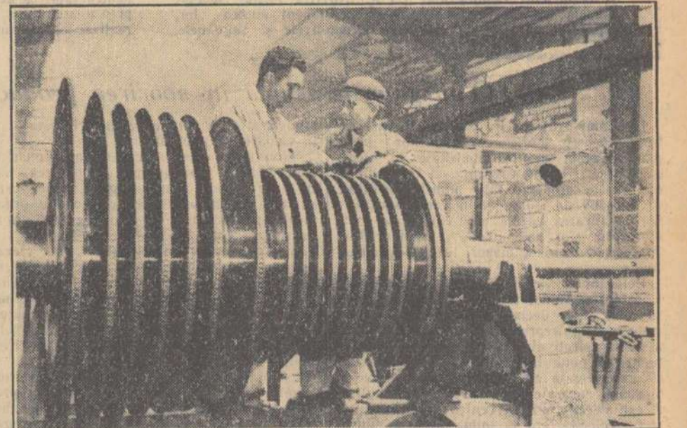
În sectorul paletaj-rotare a Combinatului metalurgic Reșița, maistrul Petro Negru explică tînrului C. Pirvu unele detalii în construcția unui rotor. Foto: P. COZIA
