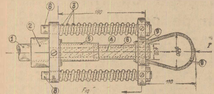
Fig. 1. Dispozitiv cu ajutorul căruia putem face această operație de curățare a cupelor de fontă pentru centrifuge (9 din fig. 1).
