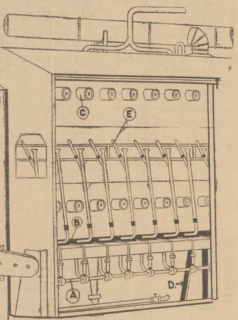
Fig. 1-a. Mașina de filat continuu a viscozei. Această mașină înlocuiește toate operațiunile necesare dela materia primă
