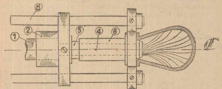
Fig. 1. Dispozitiv cu ajutorul căruia putem face această operație de curățare a cupelor de fontă pentru centrifuge (9 din fig. 1).
