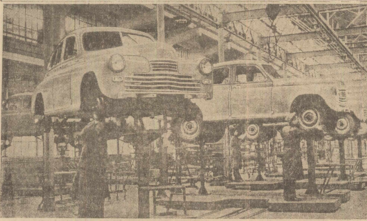
Metodele de muncă în lanț și în sistem continuu sunt practicele pe o scară largă în întreprinderile sovietice. Procesele de fabricație se automatizează la maximum. În clișeu: montajul unui automobil marca „Pobeda” (Victoria) pe linia de circulație a uzinei de automobile Molotov din orașul Gorki.
