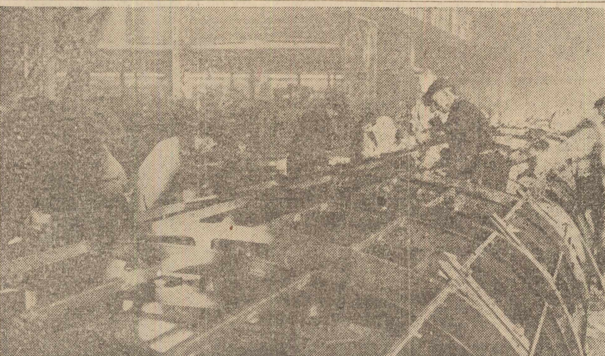
Montarea unui acoperiș de vagon de cale ferată la fabrica de vagoane și locomotive „Cegielski” din Poznań
