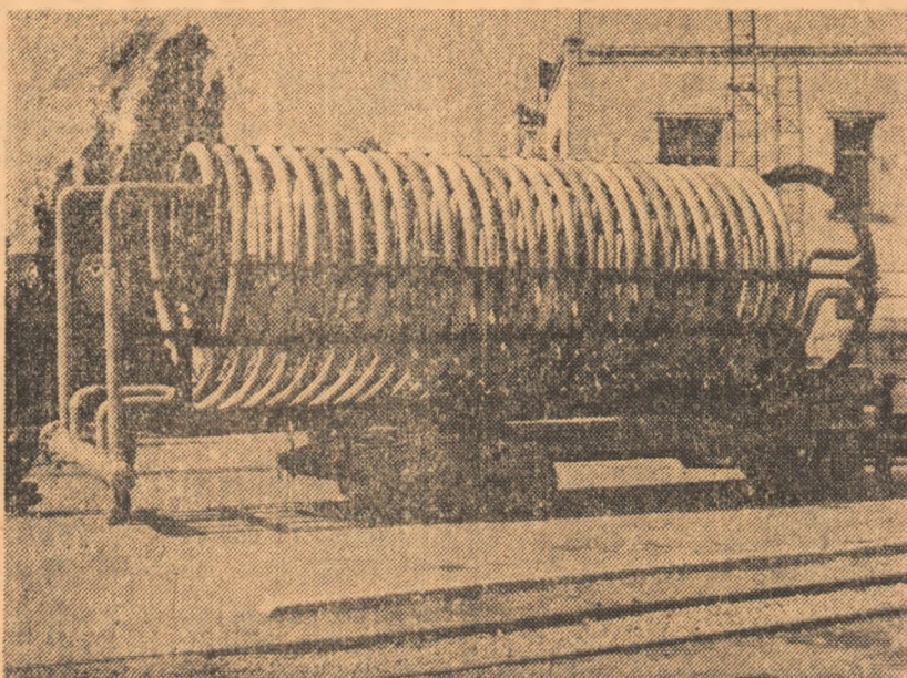
Serpentina cuptorului pentru izomerizare în industria chimică
