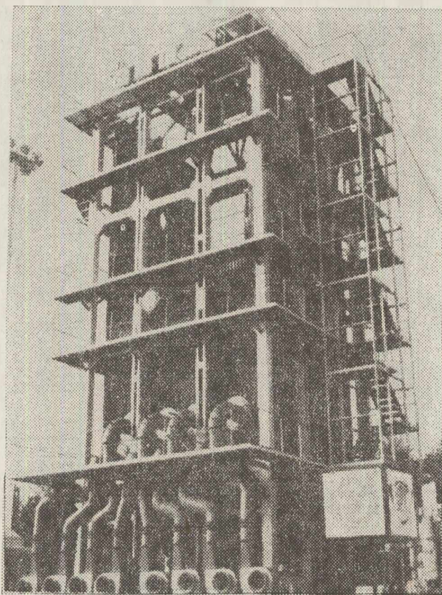
Cazan de abur 100 Gcal/h pre- zentat la una din edițiile „EREN”
