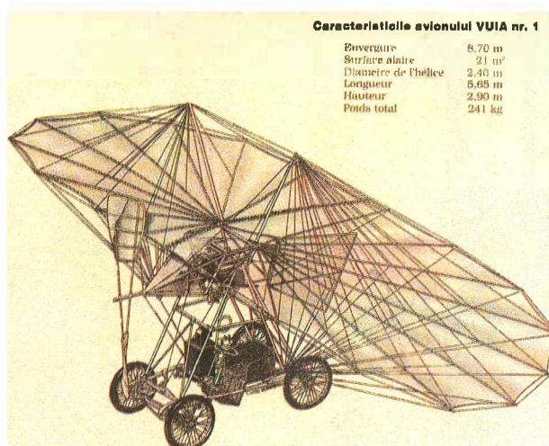
O schiță tehnică având caracteristicile aparatului VUIA-1
