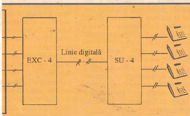
Principiul operării sistemului DS-PCM4
