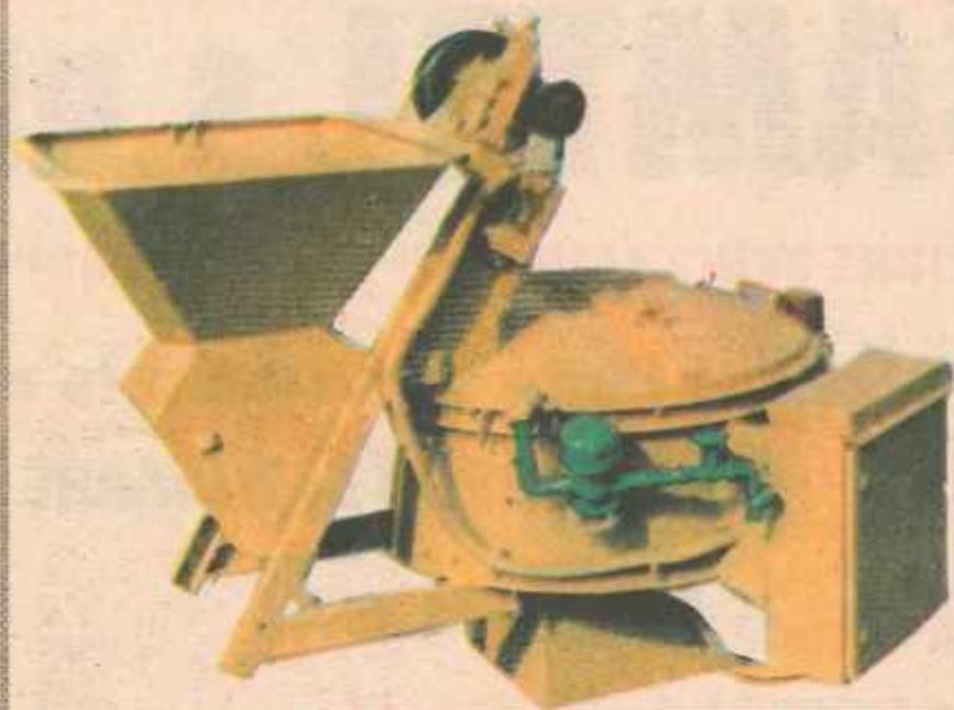
Malaxor cu amestec forțat (betoniere)
