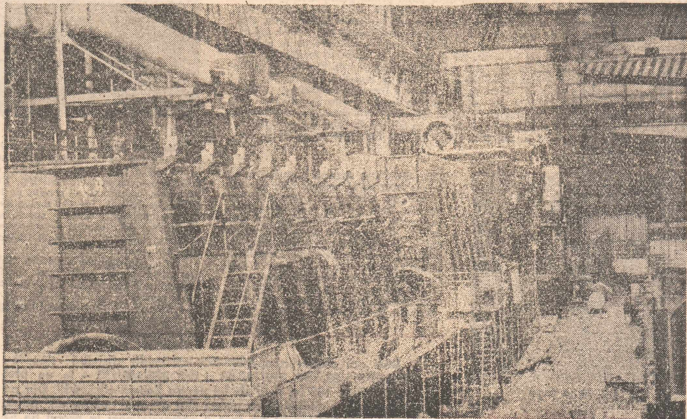
Stand de montaj al motoarelor navale
