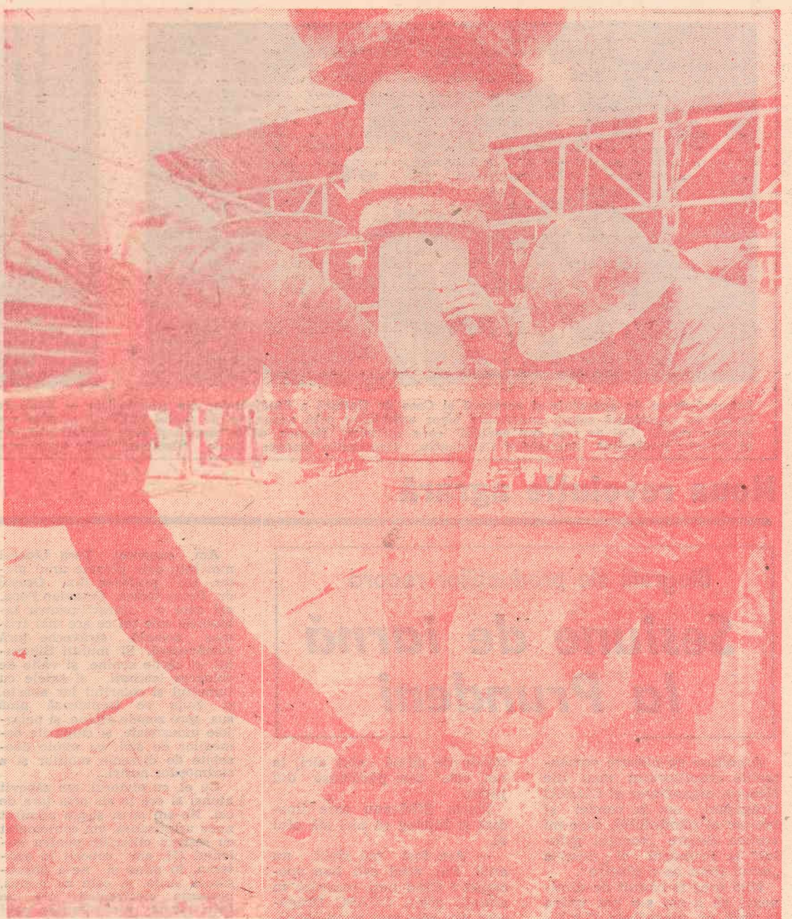
Atenție, prăjinile apasă cu forță pe sapa de foraj ce străbate erele geologice. A ajuns în Oligocen
