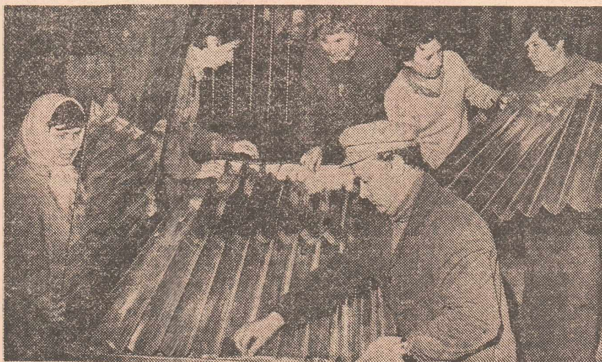
Întreprinderea de aparataje și accesorii și Casa de Cultură a Sindicatelor din Alexandria — două ferestre deschise, în acest început de an. Pe banda de montaj noile tipuri de captoare solare superioare celor anterioare prin economia de metal obținută și prin creșterea importantă a aportului energetic. La Casa de Cultură, teatrul popular repetă. Cei de față sînt oameni care au ieșit, fiecare, de la muncă și s-au întâlnit aici, de fapt, în schimbul dol, unde viața continuă în jurul citorva pasionați ai scenei: profesorul Alexandru Constantin, Constantin Mocanu, Elena Nicolescu, Tache Leonida și Alexandru Ciobanu.
